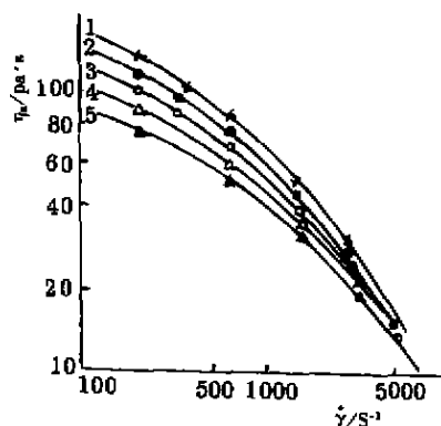
图 2 240°C PP、PU/PP 共混物的流动曲线 注:1~5 与图 1 相同
