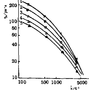
图 1 220°C PP、PU/PP 共混物的流动曲线 1 PP; 2 PU/PP=3/97; 3 PU/PP=6/94; 4 PU/PP=9/91; 5 PU/PP=12/88
