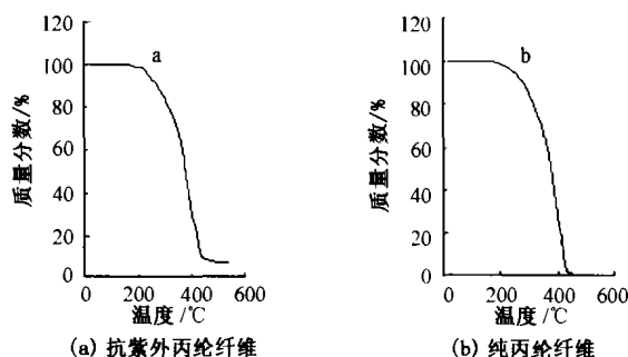
图 1 两试样的热重曲线
